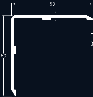
HA 206 0.426 Kg/m
