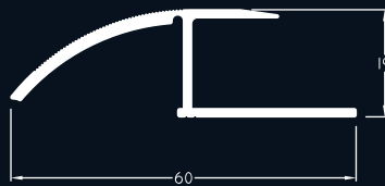
HA 1421 0.399 Kg/m
