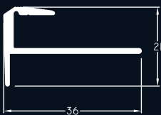
HA 2907 0.258 Kg/m
