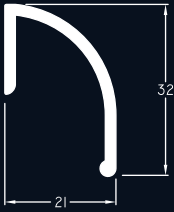
HA 534 0.317 Kg/m
