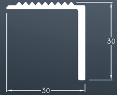
HA 2878 0.325 Kg/m
