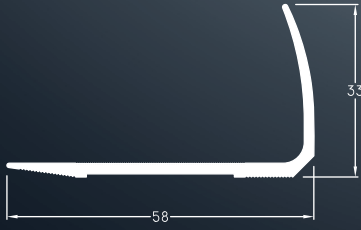
HA 2850 0.432 Kg/m
